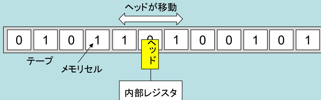
チューリング・マシンの原理図
