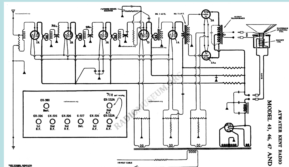
回路図(RADIOMUSEUM USA)
